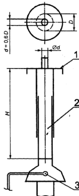
Рисунок И.10 — Устройство для определения гидравлического сопротивления
