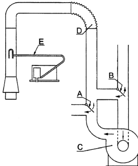
Рисунок И.4 — Устройство для отбора проб и измерения температуры продуктов сгорания для дымохода диаметром, не превышающим 100 мм
