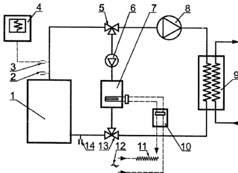
Рисунок И.8 — Испытательный стенд для определения КПД
