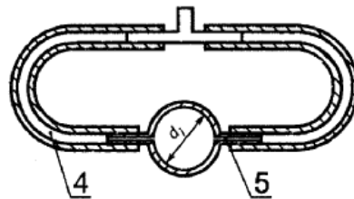
Деталь X (секция развернута на 90°)
