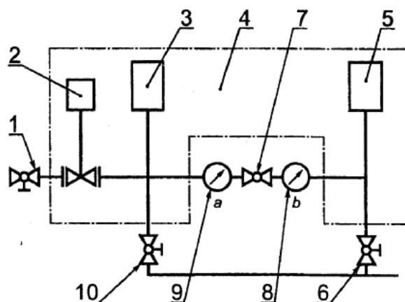
Рисунок И.6 — Устройство для проверки герметичности газового тракта
